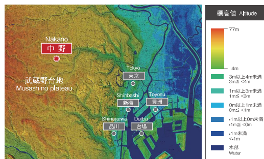
地盤イメージ図
