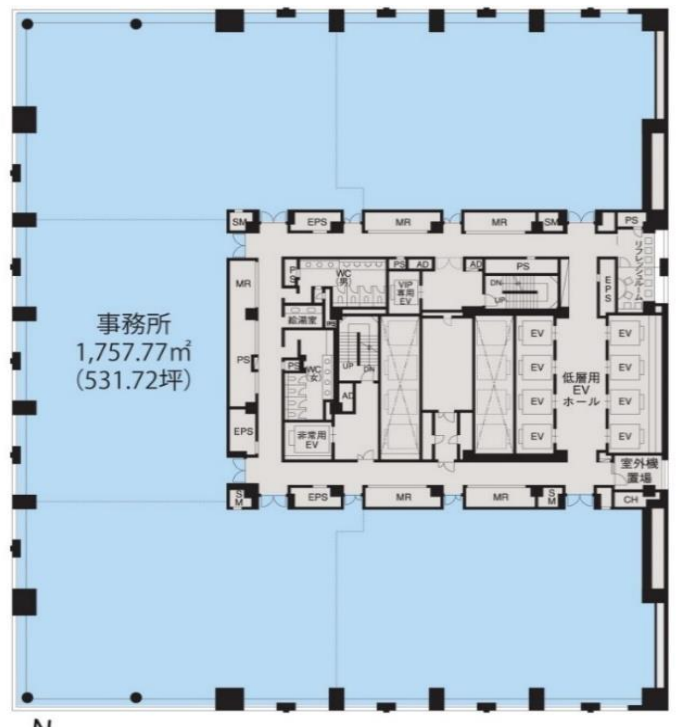
10階
