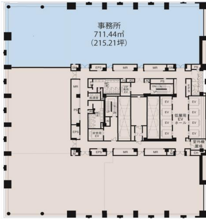
9階・17階
